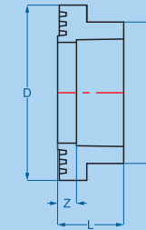
VAI BÍCH KÉP / Flange steel body
